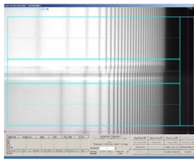
2段強化ガラス
