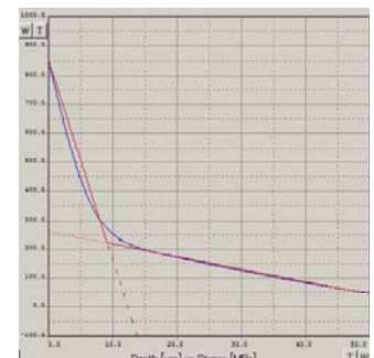
断面応力分布 (例: 2段強化ガラス)
